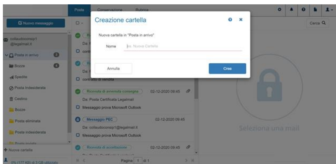
FIGURA 4 CONFERMA CREAZIONE
